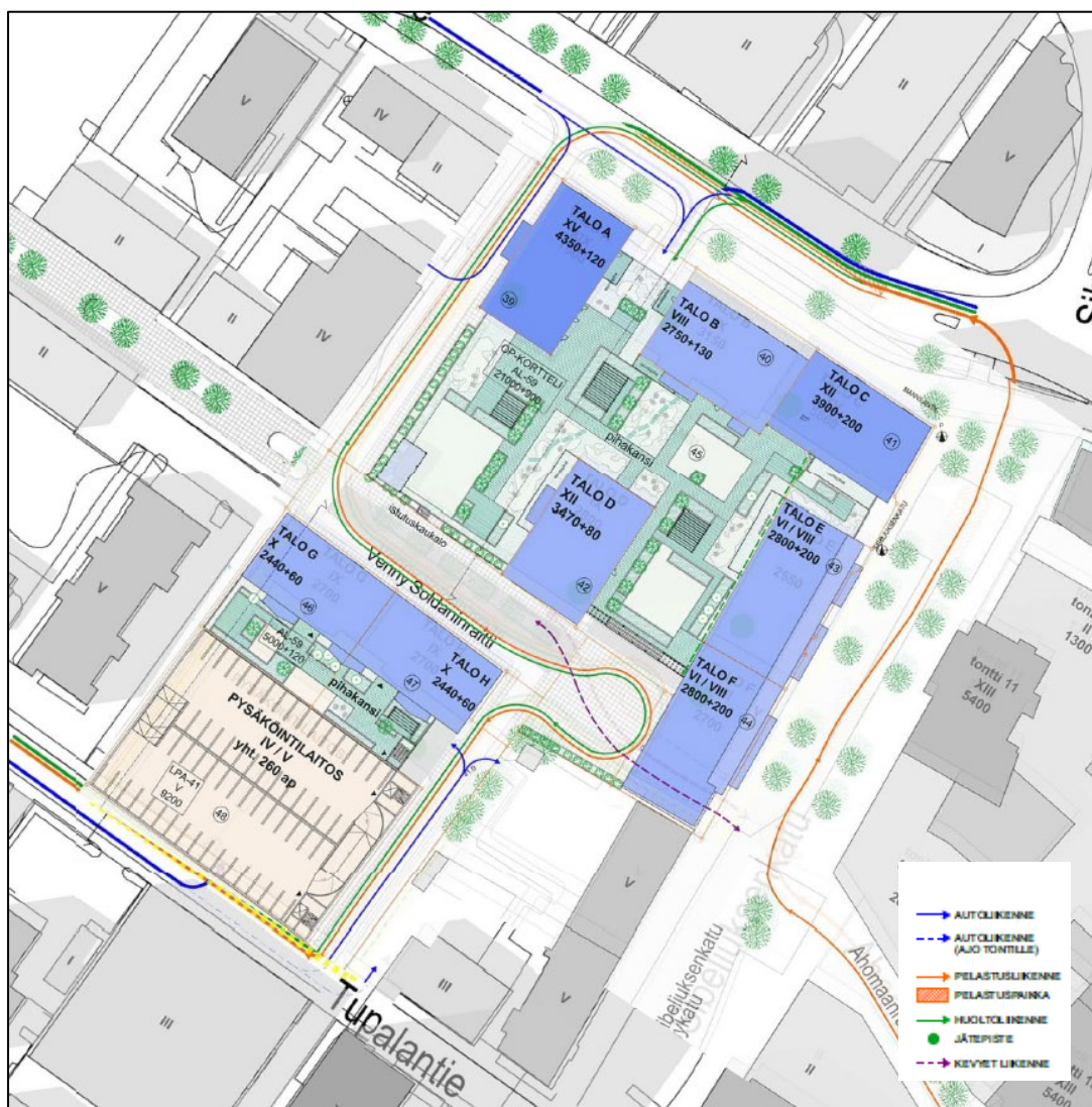
Kuva 4. YIT Rakennus Oy:n laadittama alustava viitesuunnitelma, Arco Architecture Company Oy, 05.03.2024.
